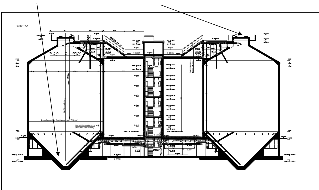
Faulbehälter Ost und West (Schnitt)
