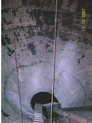
Prüfung des Behälterbodens
