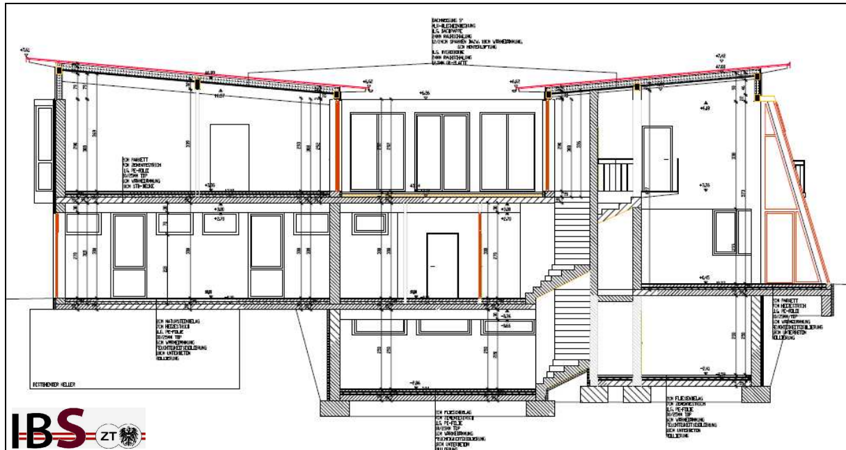
Gebäudeschnitt (Einreichprojekt)
