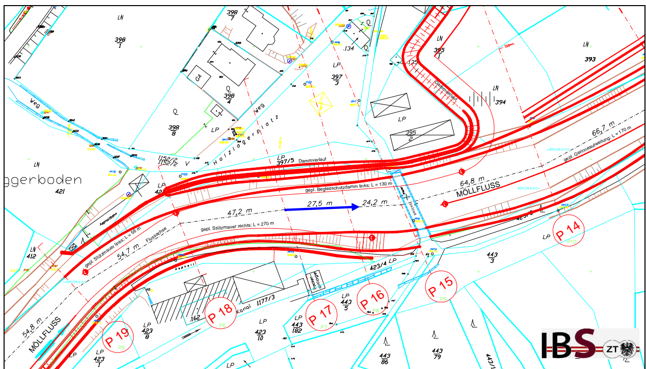
Lageplan der Schutzmaßnahmen mit Mauern rechtsseitig und Erdschüttdämmen linksufrig
